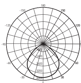
PFL-V 100w
